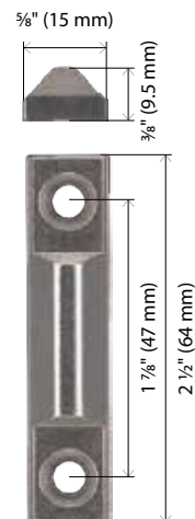
No DXAS224* Gâche inférieure En option pour DX2PV et DX2PW. (Grade2) P
