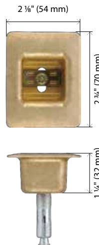
N° DXAS227 / 227F Gâche inférieure Standard pour DX2PV/FV, DX2PC/FC, DX2PW/FW. P 🔥
