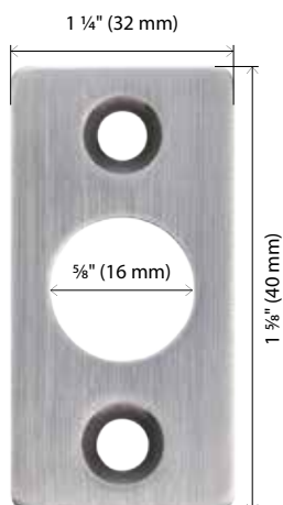
No DXAS225* Gâche inférieure Pour DX2PV, DX2PC, DX2PW avec pêne à coulisse ronde. (Grade2) P
