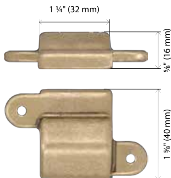
N° DXAS216 Gâche supérieure Standard pour DX2PC/FC. P 🔥
