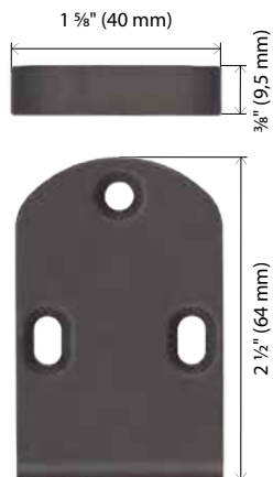
N° DXAS215* Gâche supérieure Pour traverse plate DX2PV/FV, DX2PW/FW. P 🔥
