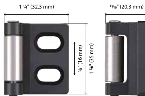
N° DXAS203 Gâche supérieure Pour DX2PV, DX2PW. P
